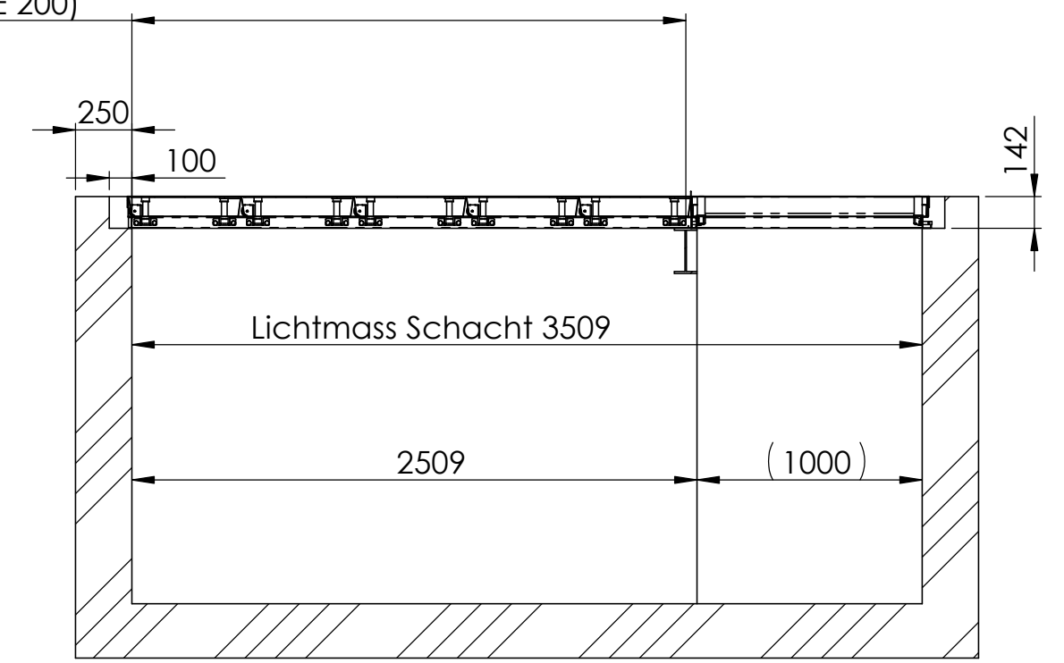
SCHNITT B-B MABSTAB 1 : 30
