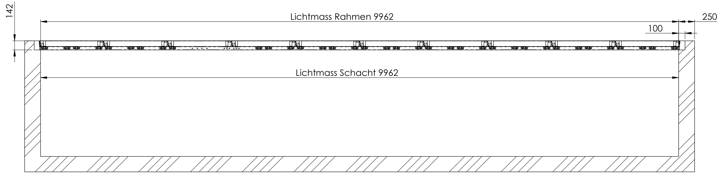
SCHNITT A-A MABSTAB 1 : 30
