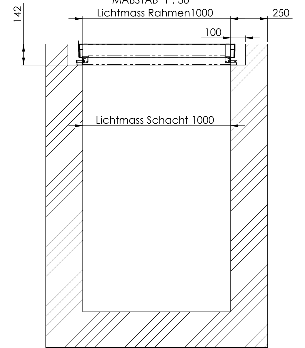
SCHNITT C-C MABSTAB 1 : 15
